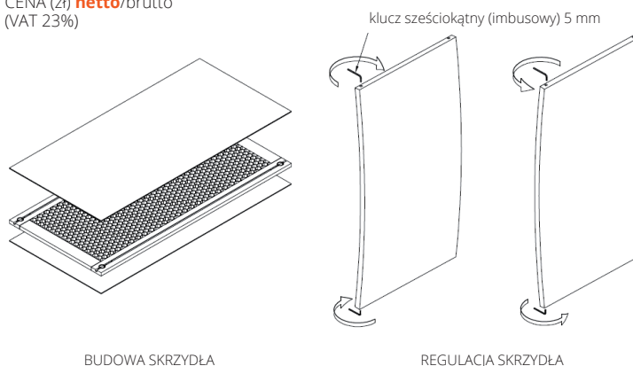
BUDOWA SKRZYDŁA
