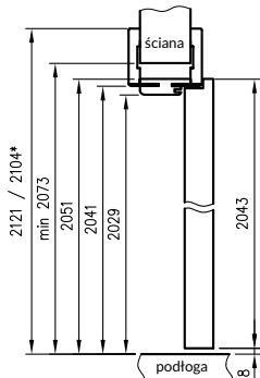
Przekrój pionowy drzwi przylgowych z OR
