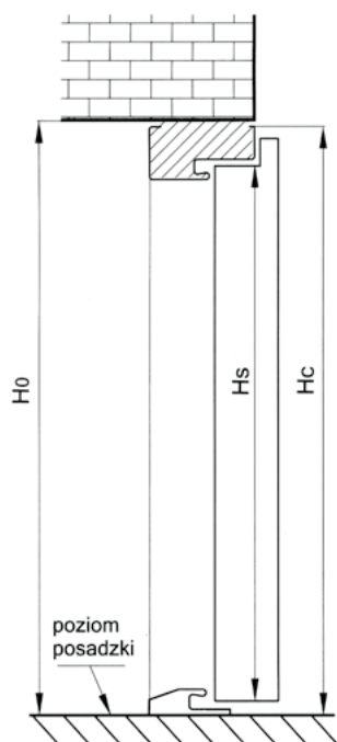
Ościeżnica TERMO do PREMIUM i EXPERT 64
