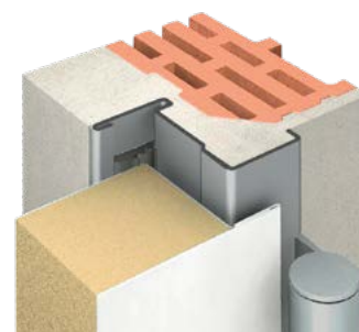
OŚCIEŻNICA PROFIL 375 M
