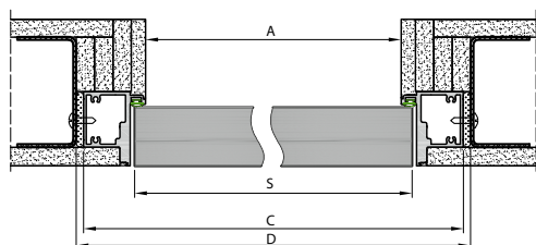
Przekrój pionowy drzwi Sara Eco 2
